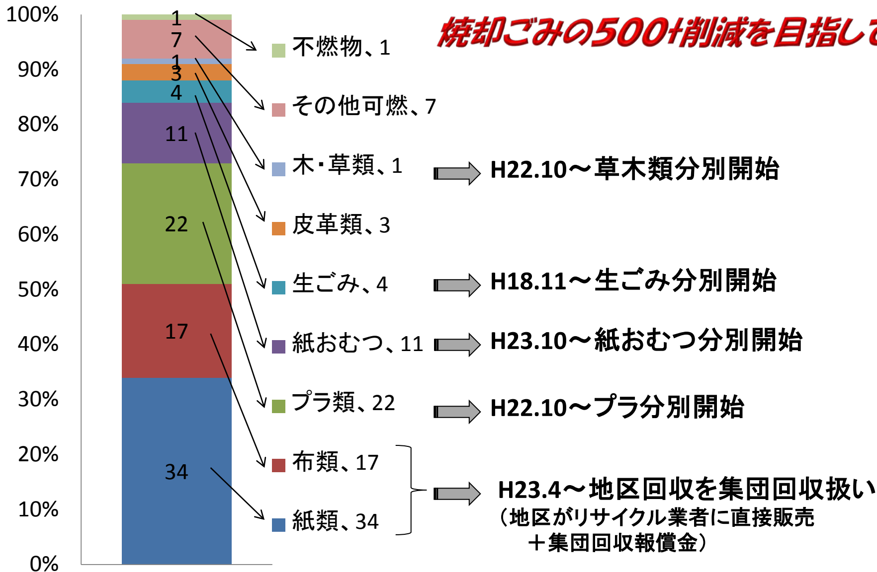
H20燃やすごみの 組成(重量比)
